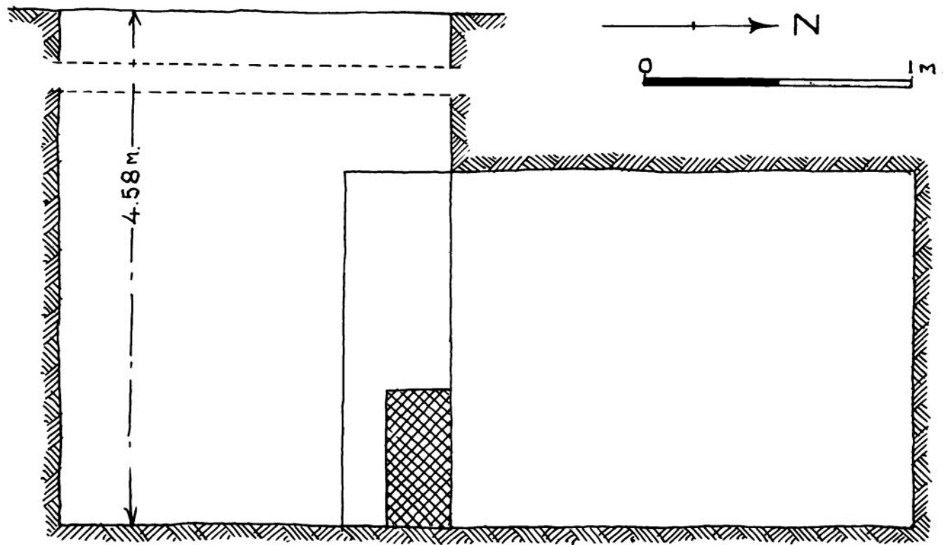
Sec. A-B
