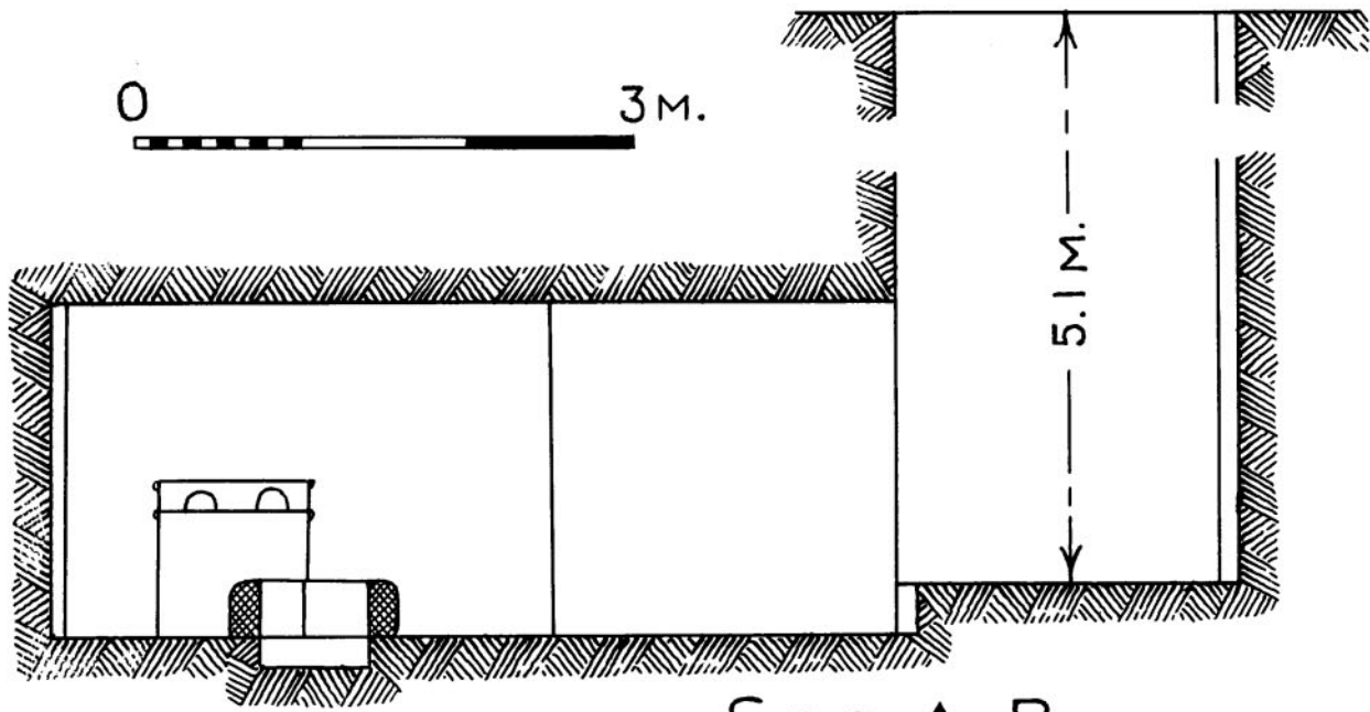
Sec. A-B
